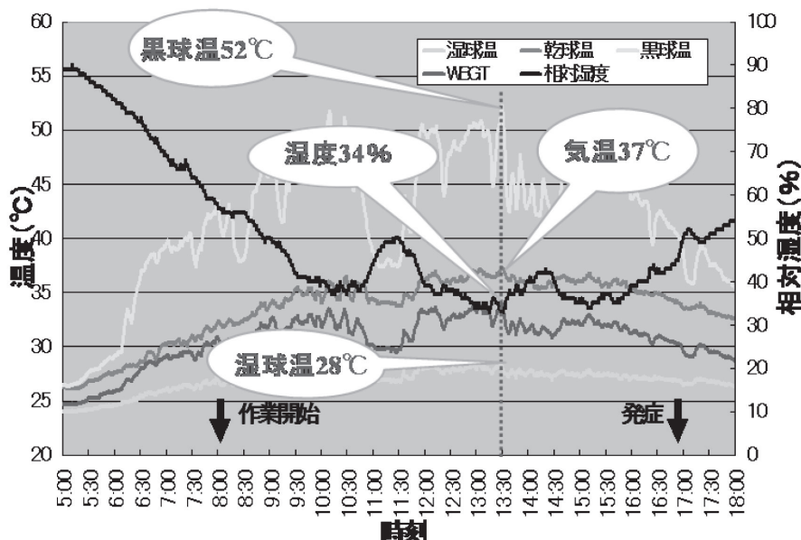
図Ⅳ－3 熱中症災害発生日の温熱環境条件の日内変動（澤田：2013）
