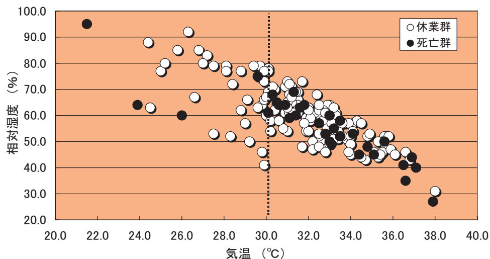
図Ⅳ－１ 屋外作業での熱中症発生時における気温と湿度（澤田、福田：2000）
